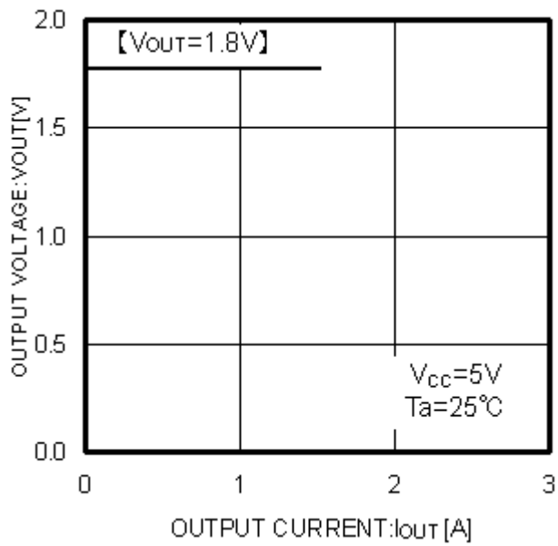
Fig.6 Iout-Vout
