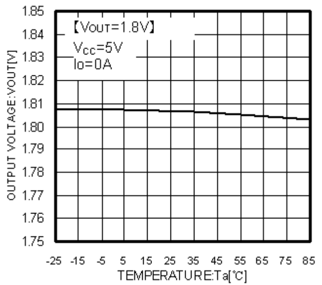
Fig.7 Ta-Vout
