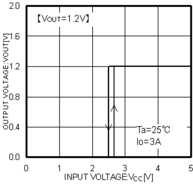
Fig.4 Vcc - VOUT
