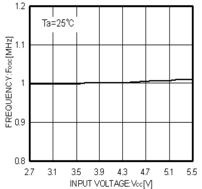
Fig.13 V_{cc} - F_{osc}
