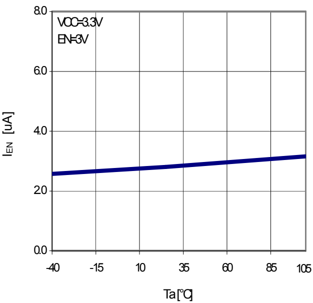
Fig.24 T_a - I_{EN}
