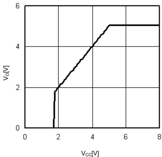
Fig.15 V_{CC}-V_O ( I_O=0\text{mA} )
