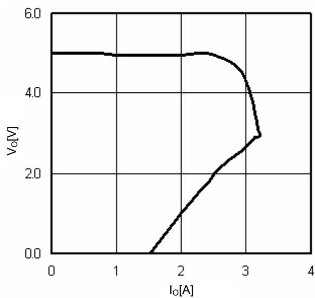
Fig.17 OCP
