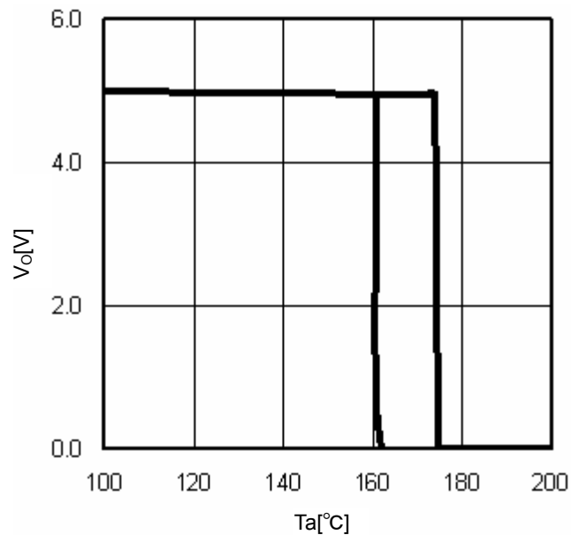
Fig.16 TSD ( I_O=0\text{mA} )
