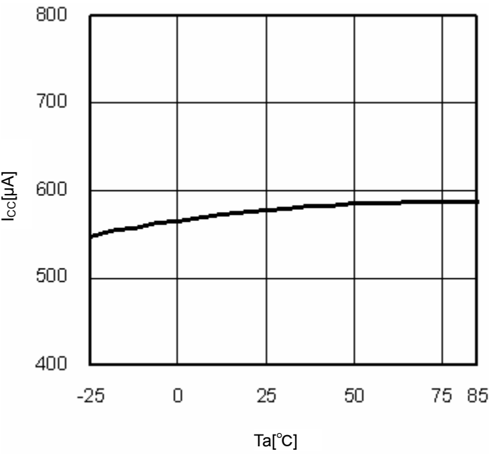
Fig.10 T_a-I_{cc}
