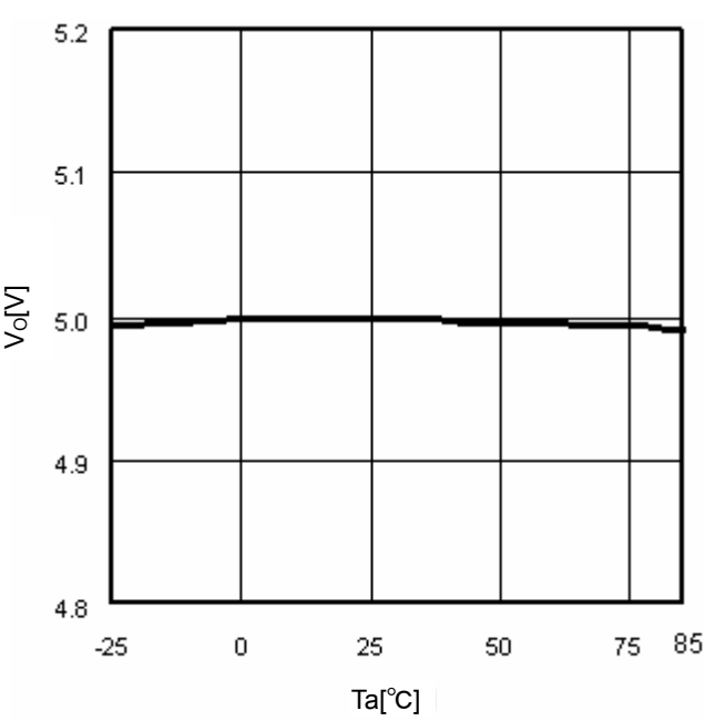
Fig.9 T_a-V_O ( I_o=0mA )
