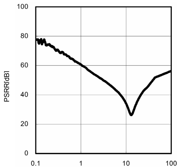
Fig.33 PSRR( I_O=0mA )
