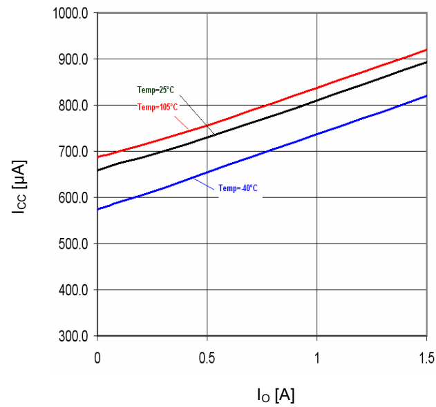
Fig.32 I_O - I_{CC}
