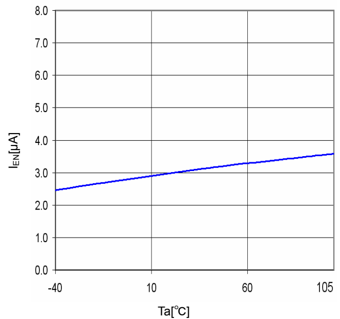
Fig.24 T_a - I_{EN}
