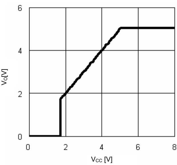
Fig.15 V_{CC}-V_O ( I_O=0mA )
