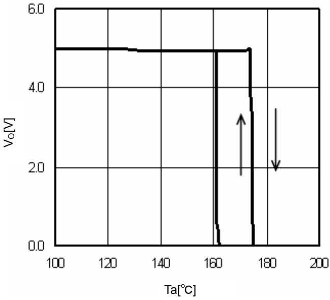
Fig.16 TSD ( I_O=0mA )
