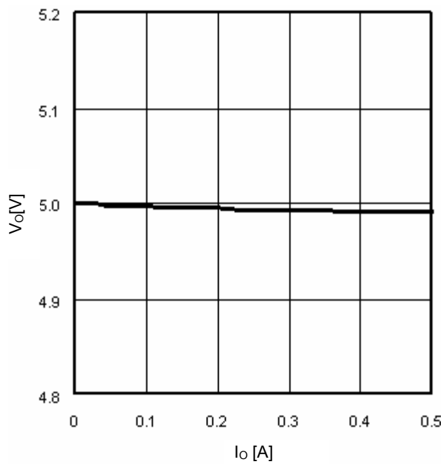
Fig.13 I_O - V_O
