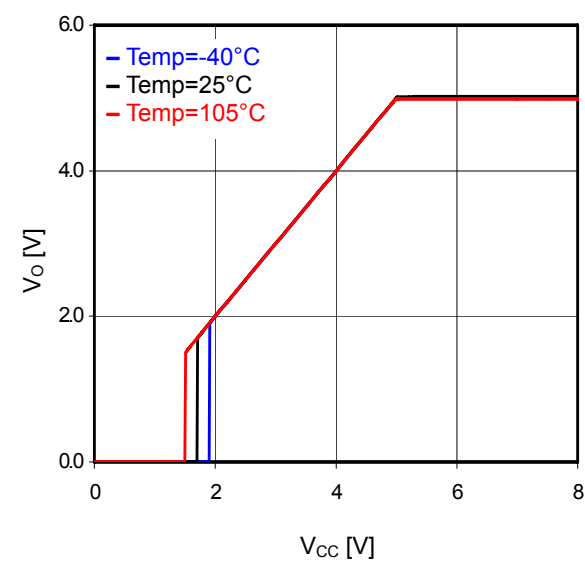
Fig. 27 V_{CC}-V_O ( I_O=0mA )
