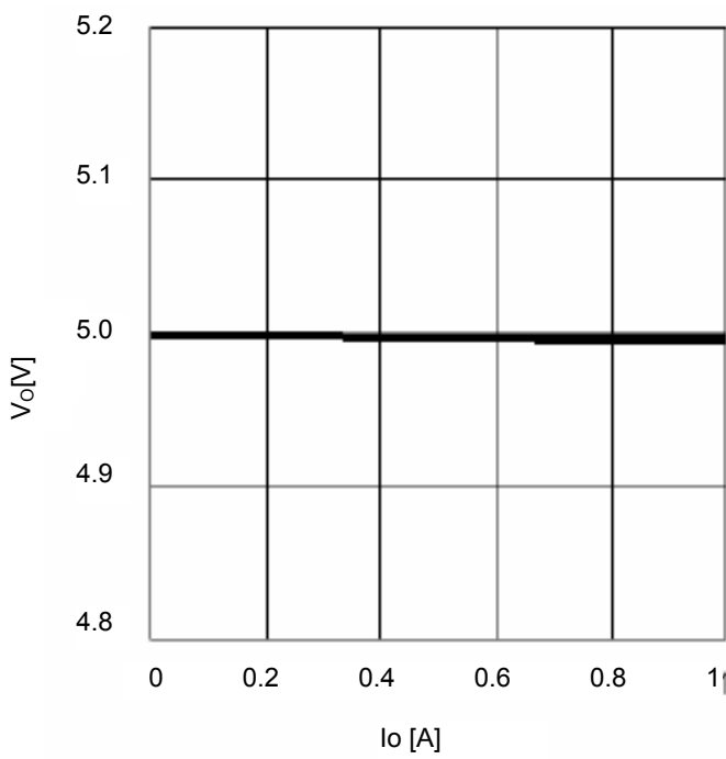
Fig.25 I_O - V_O
