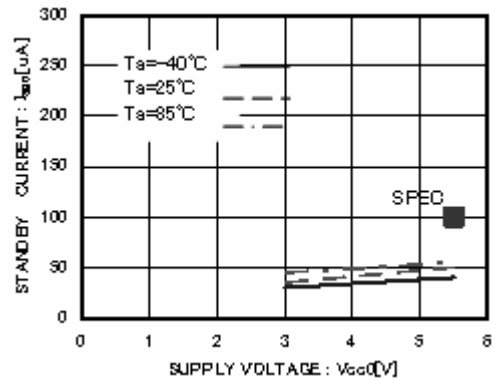
Figure 21. Standby Current0 I_{St0}
