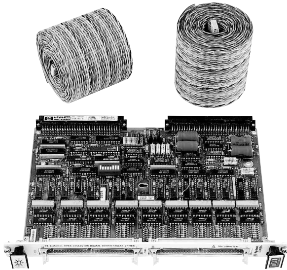
Agilent E1339A
