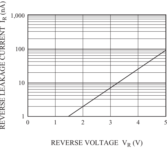
I_R - V_R
