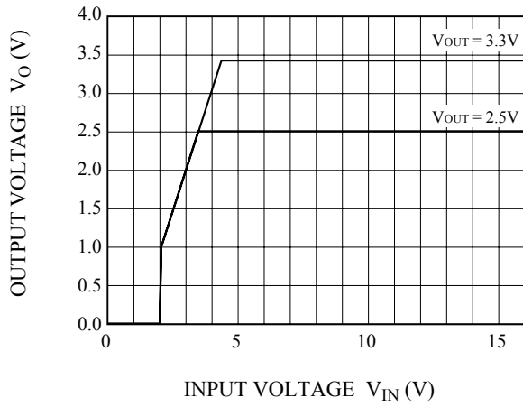
Fig. 3 V_{OUT} - V_{IN}
