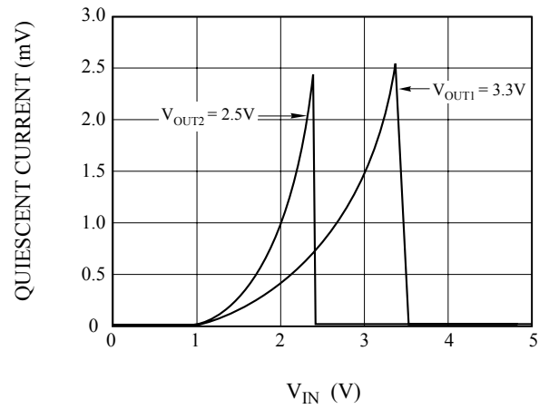
Fig. 4 I_q - V_{IN}
