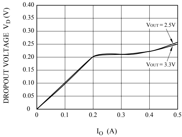
Fig. 5 V_D - I_{OUT}
