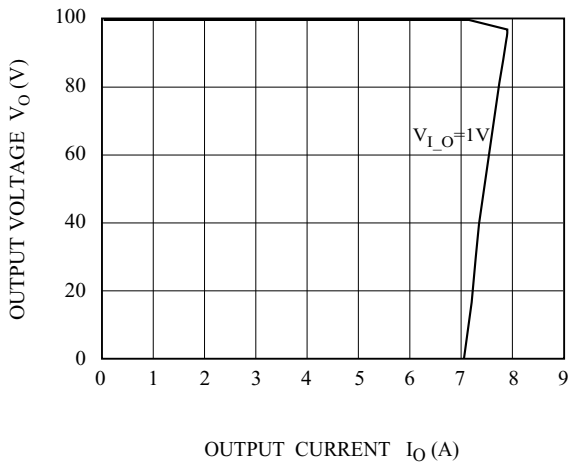
Fig. 4 I_O - V_O
