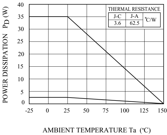
Fig. 12 P_D - T_a (FP-Type D2PAK-5)
