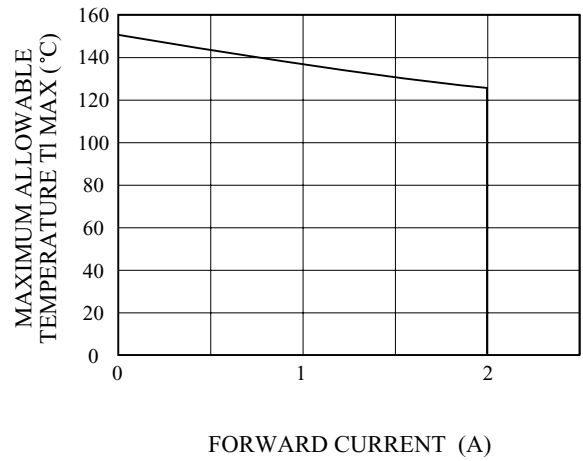
T_l - I_F
