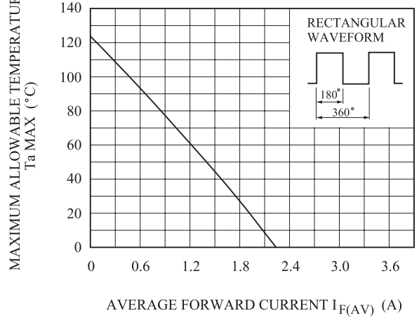
T_a - I_{F(AV)}
