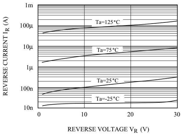
I_R - V_R
