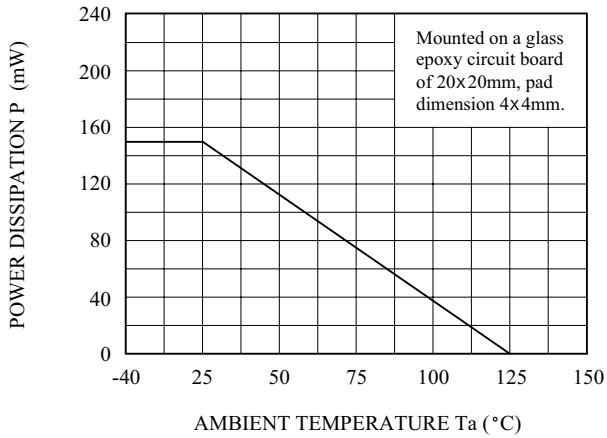
P - T_a
