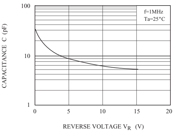
C - V_R
