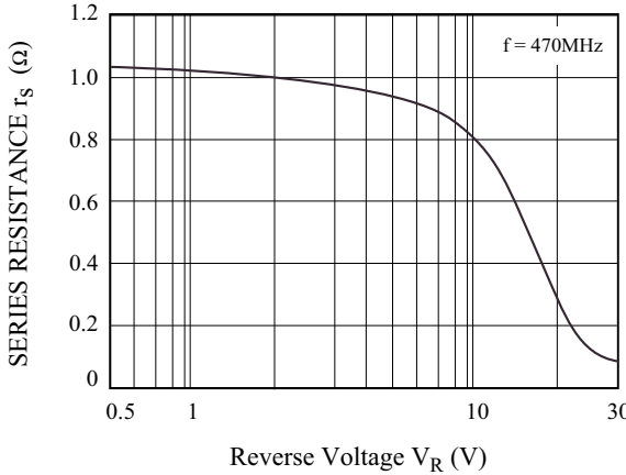
r_s - V_R
