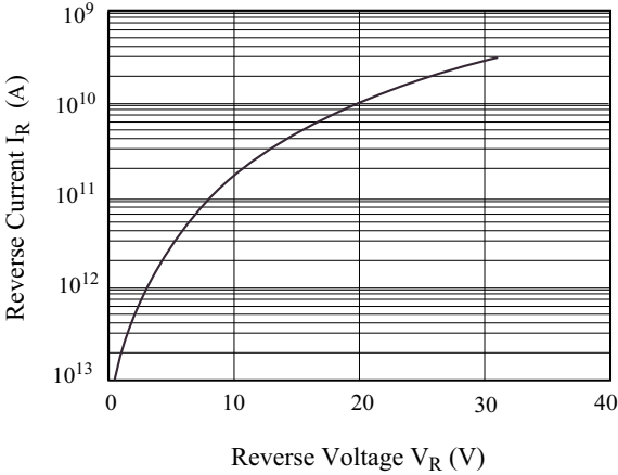
I_R - V_R
