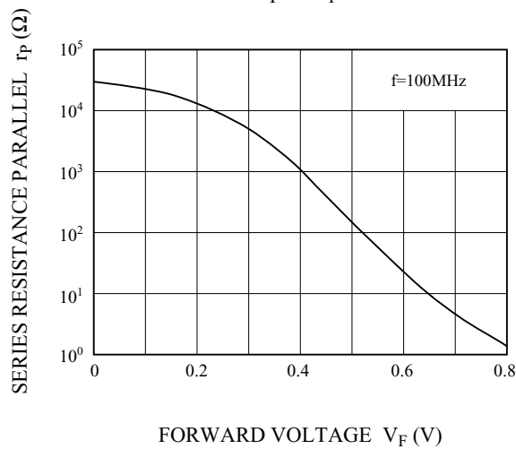
r_p - V_F
