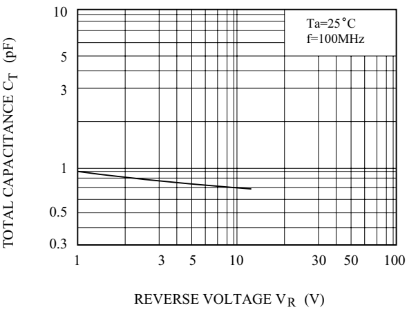
C_T - V_R
