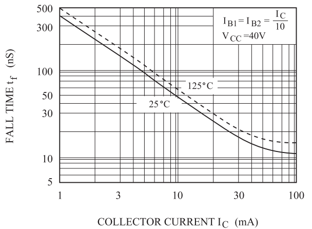
t_f - I_C
