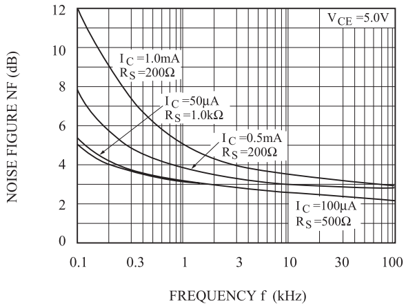
NF - f
