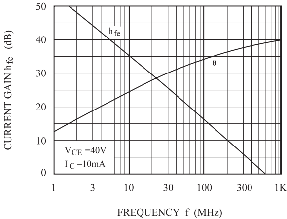
h_{fe} - f
