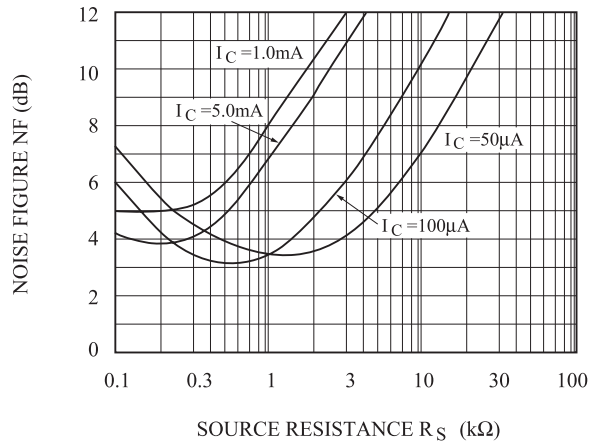
NF - R_S
