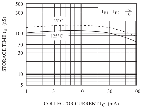
t_s - I_C
