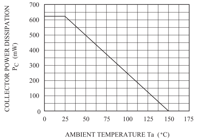
P_c - T_a
