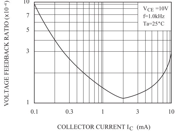
h_{re} - I_C
