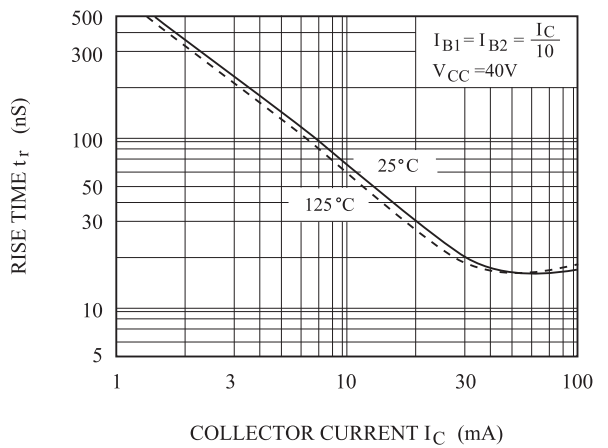
t_r - I_C
