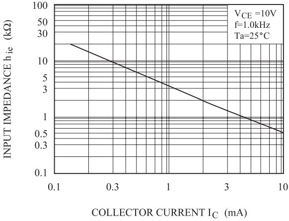
h_{ie} - I_C
