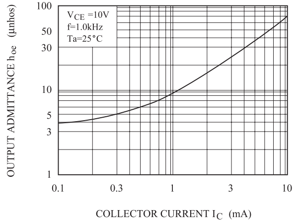
h_{oe} - I_C
