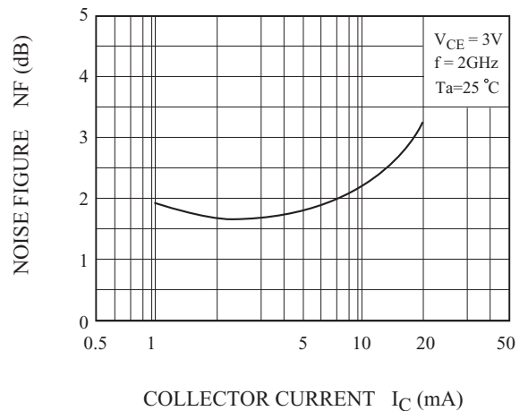
NF - I_C
