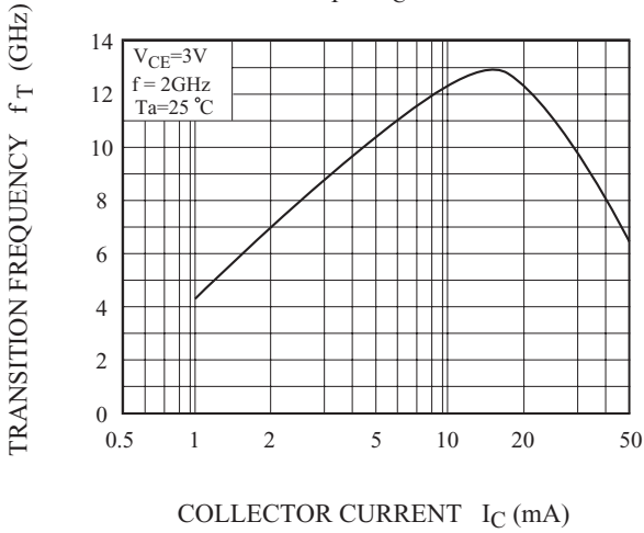
f_T - I_C
