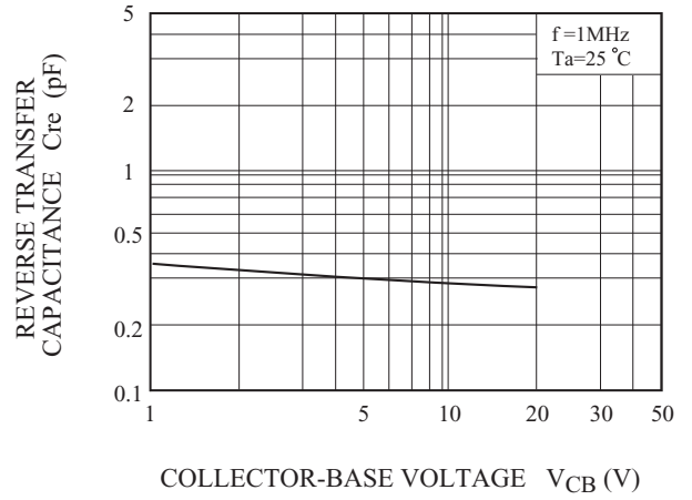
C_{re} - V_{CB}
