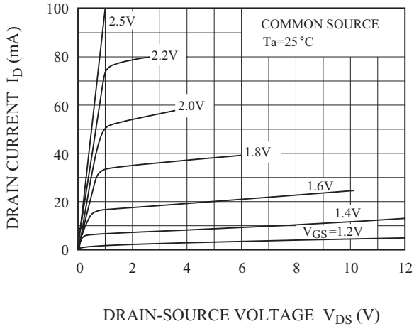
I_D - V_{DS}
