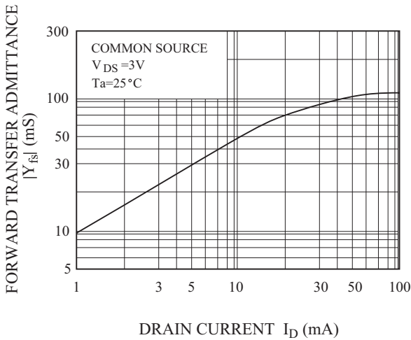
|Y_{fs}| - I_D
