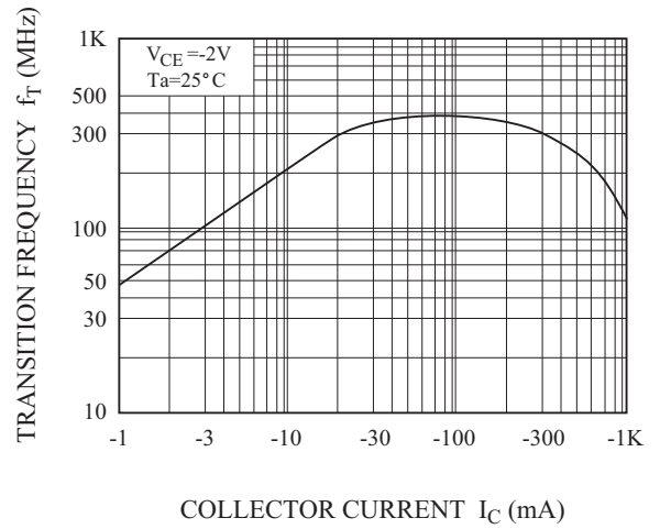
f_T - I_C
