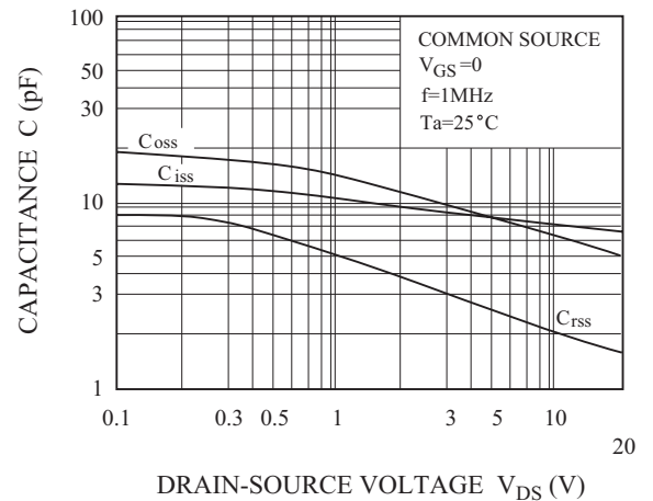
C - V_{DS}
