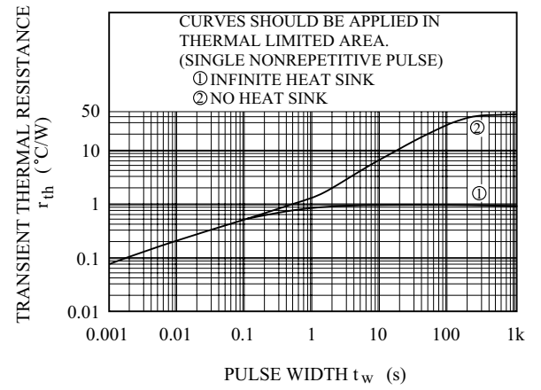
r_{th} - t_w
