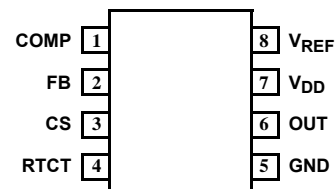
ISL78840ASEH, ISL78841ASEH, ISL78843ASEH, ISL78845ASEH (8 LD SBDIP) TOP VIEW
