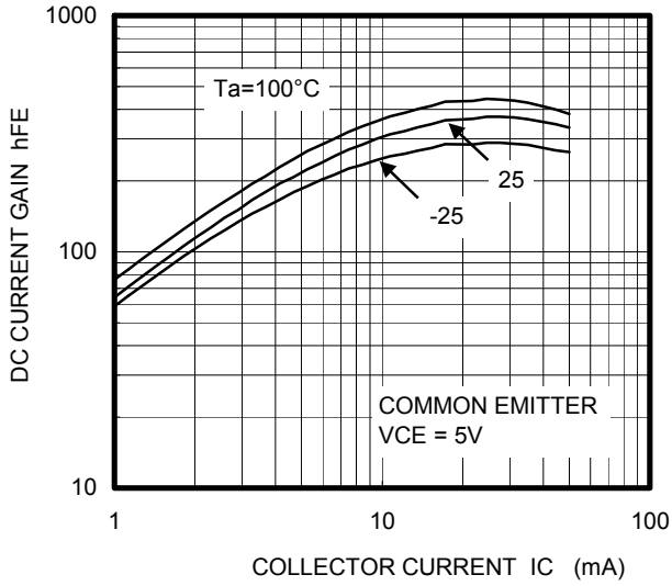
hFE - IC
