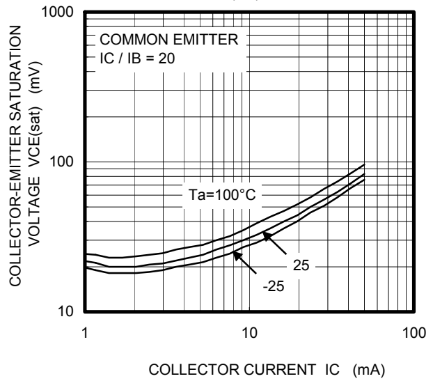
VCE(sat) - IC
