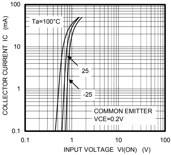
IC - VI(ON)
