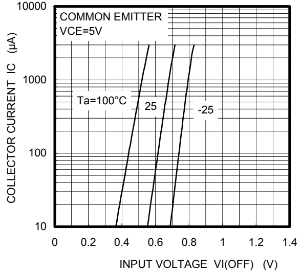
IC - VI(OFF)
