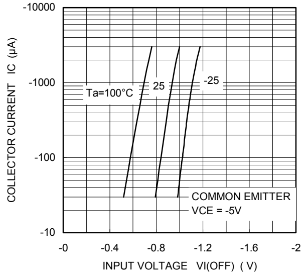
IC - VI(OFF)
