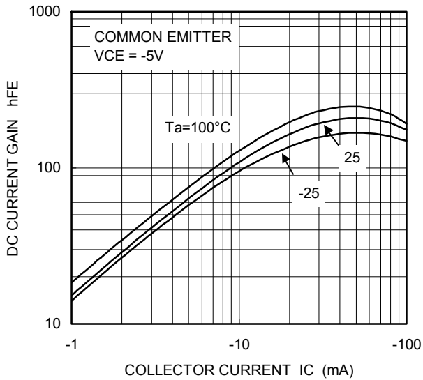
hFE - IC
