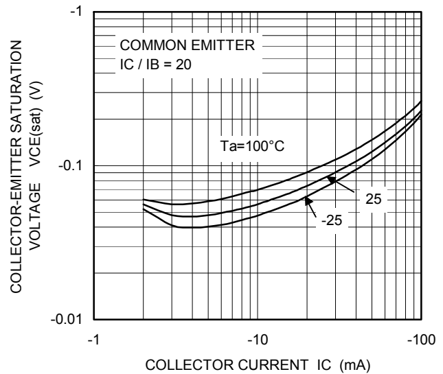
VCE(sat) - IC
