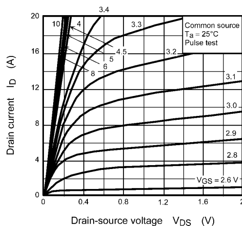
Fig. 8.2 I_D - V_{DS}
