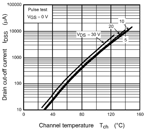
Fig. 8.16 I_{DSS} - T_{ch}
