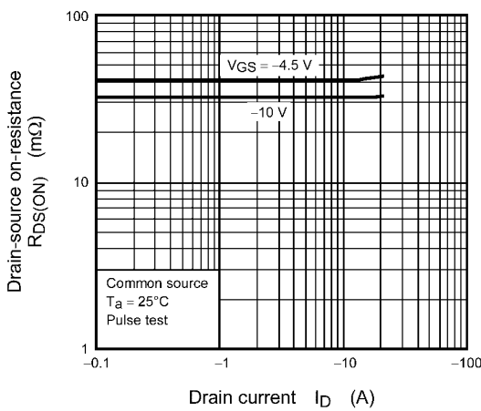
Fig. 8.1.5 R_{DS(ON)} - I_D
