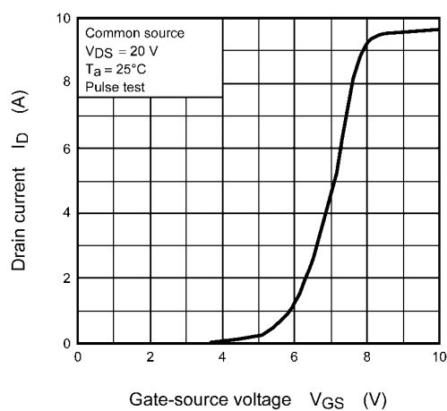
Fig. 8.3 I_D - V_{GS}
