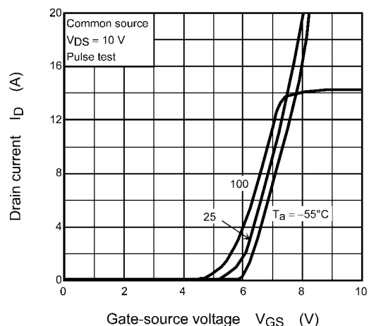
Fig. 8.3 I_D - V_{GS}
