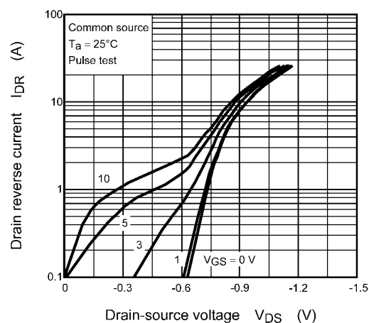
Fig. 8.8 I_{DR} - V_{DS}
