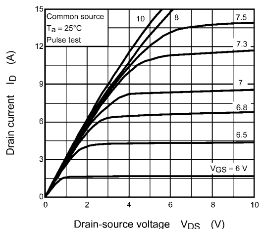
Fig. 8.1 I_D - V_{DS}
