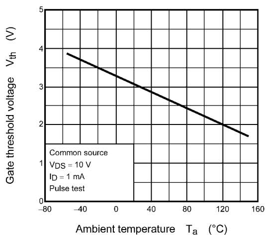
Fig. 8.10 V_{th} - T_a
