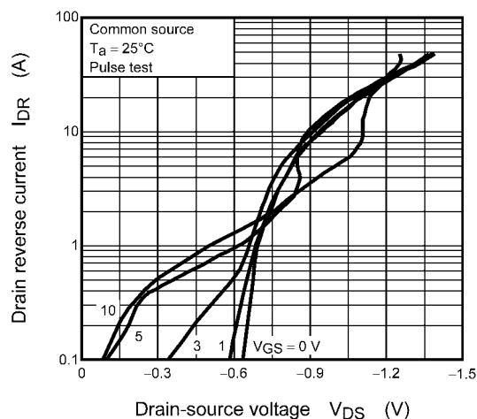
Fig. 8.8 I_{DR} - V_{DS}
