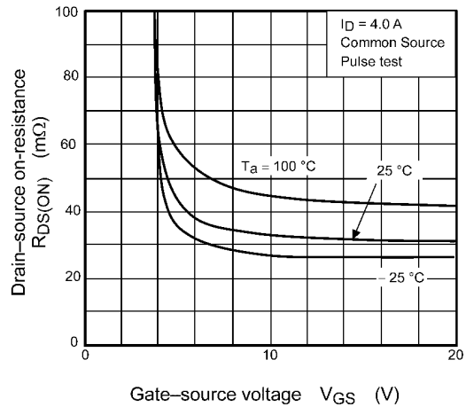
Fig. 7.4 R_{DS(ON)} - V_{GS}
