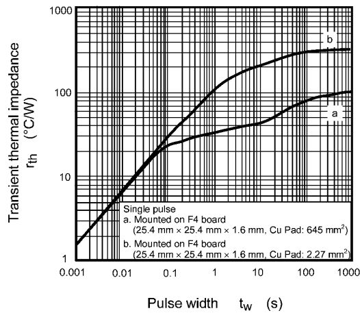
Fig. 7.13 r_{th} - t_w
