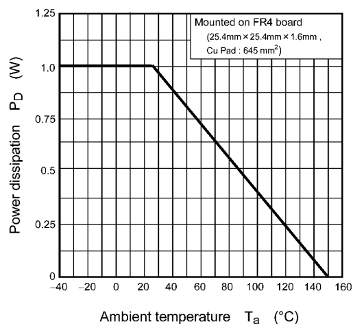
Fig. 7.13 P_D - T_a
