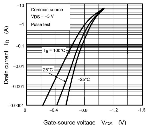
Fig. 7.2 I_D - V_{GS}
