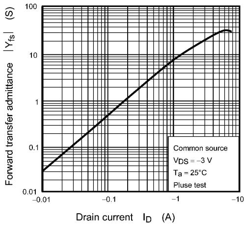
Fig. 7.7 |Y_{fs}| - I_D
