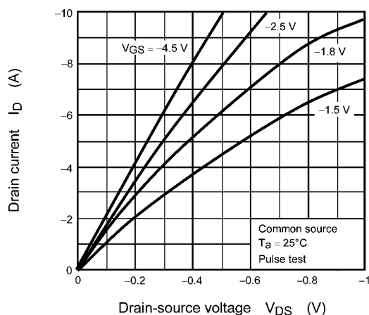
Fig. 7.1 I_D - V_{DS}
