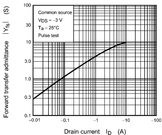
Fig. 7.8 |Y_{fs}| - I_D
