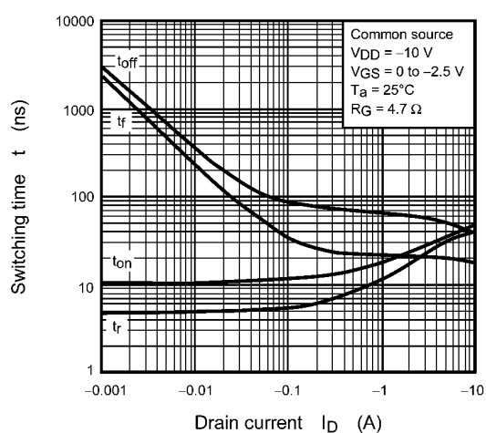
Fig. 7.11 t - I_D
