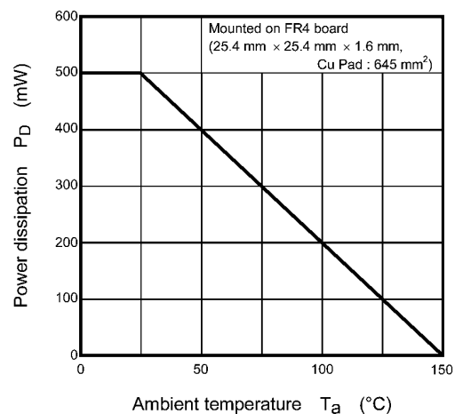
Fig. 7.14 P_D - T_a
