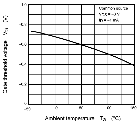
Fig. 7.7 V_{th} - T_a
