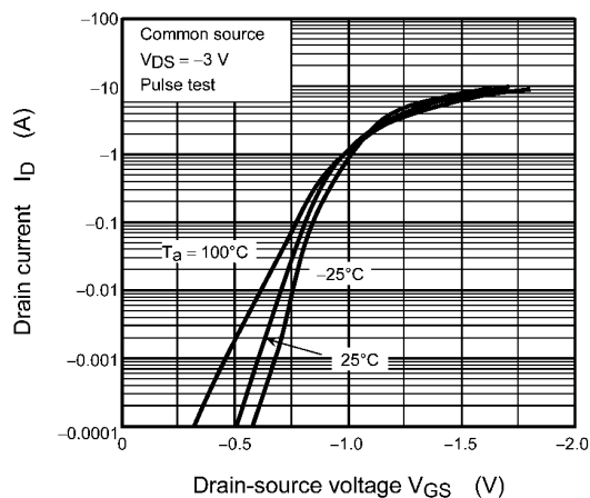
Fig. 7.2 I_D - V_{GS}
