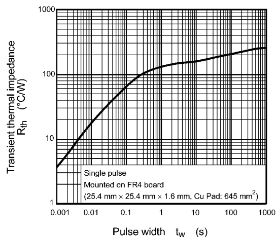
Fig. 7.13 r_{th} - t_w
