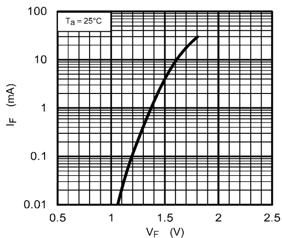
Fig. 12.1.3 I_F - V_F
