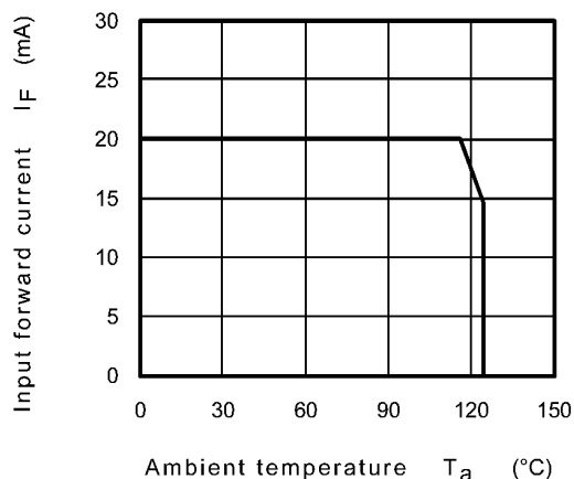
Fig. 12.2.2 I_F - T_a
