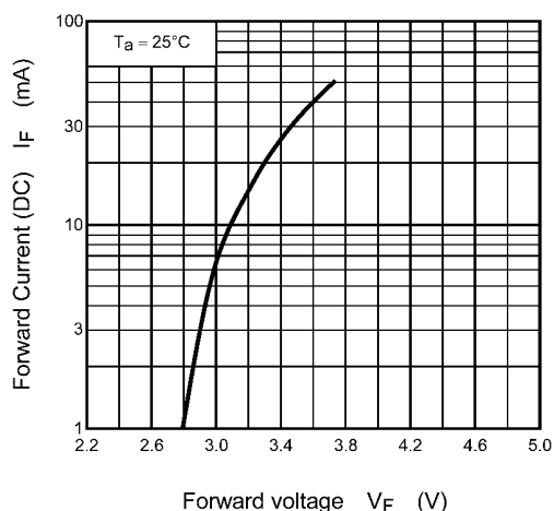
Fig. 8.1 I_F - V_F
