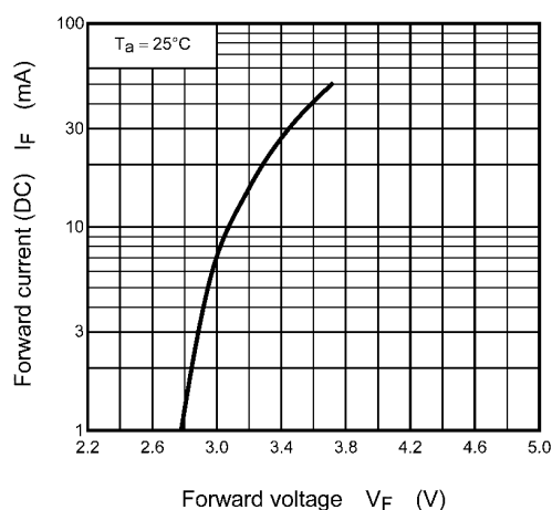
Fig. 8.1 I_F - V_F
