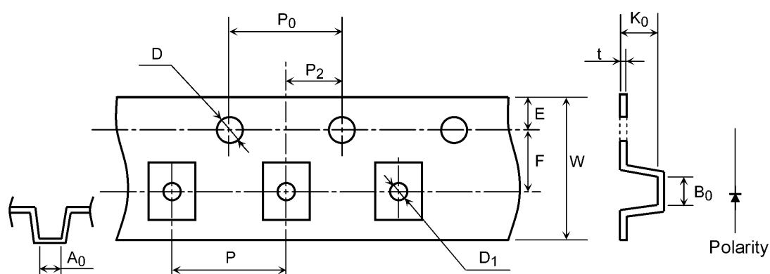
Fig. 12.2.1 Tape Dimensions
