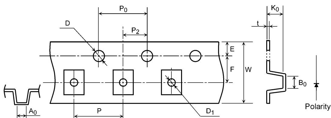
Fig. 12.2.1 Tape Dimensions
