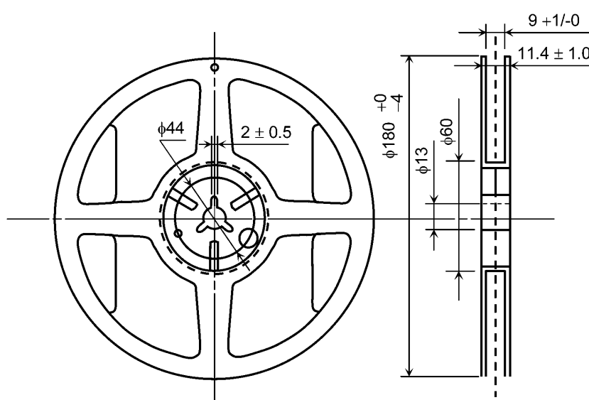
Fig. 12.3.1.1 Reel Dimensions
