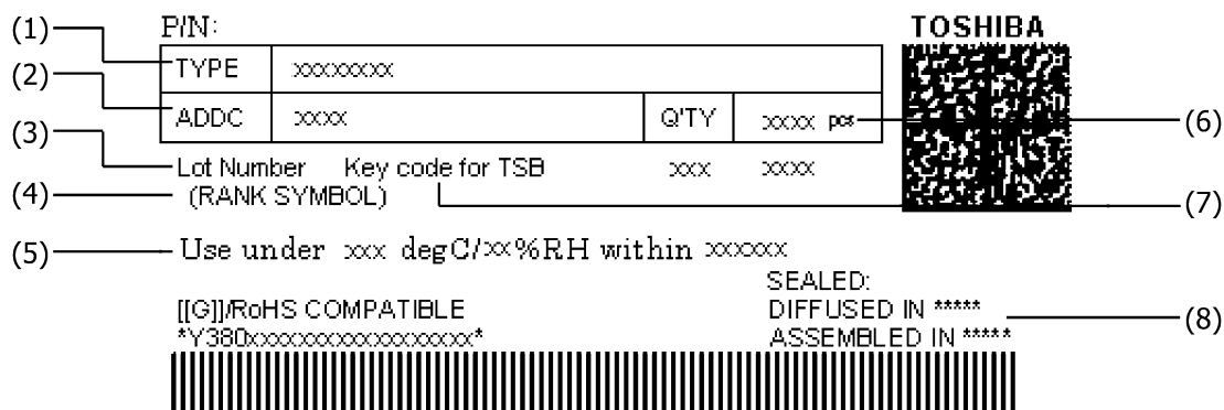
Fig. 12.5.1.1 Label Example
