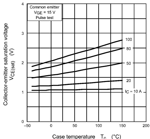
Fig. 8.4 V_{CE(sat)} - T_C
