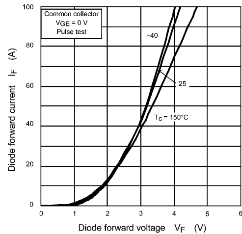
Fig. 8.10 I_F - V_F
