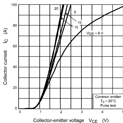
Fig. 8.2 I_C - V_{CE}
