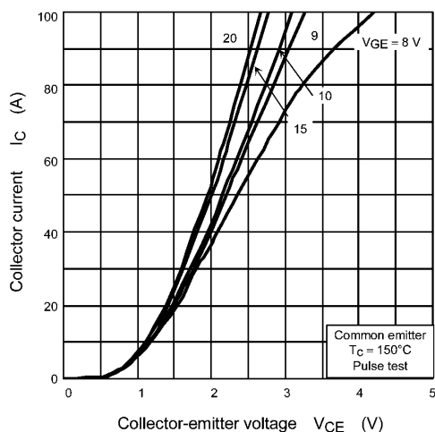
Fig. 8.3 I_C - V_{CE}
