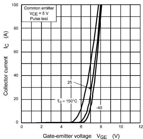
Fig. 8.5 I_C - V_{GE}
