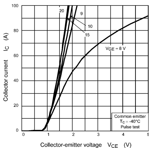
Fig. 8.1 I_C - V_{CE}
