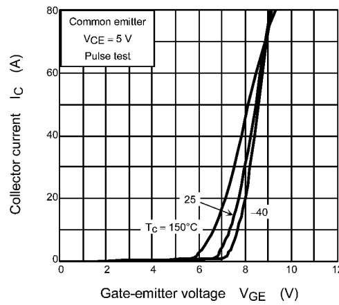
Fig. 8.6 I_C - V_{GE}
