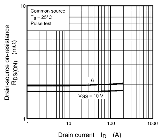
Fig. 9.5 R_{DS(ON)} - I_D
