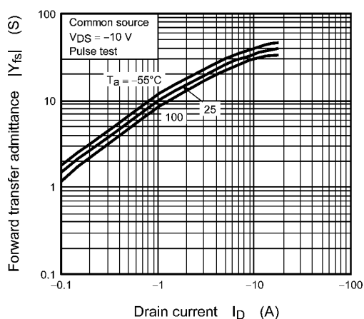
Fig. 8.5 |Y_{fs}| - I_D
