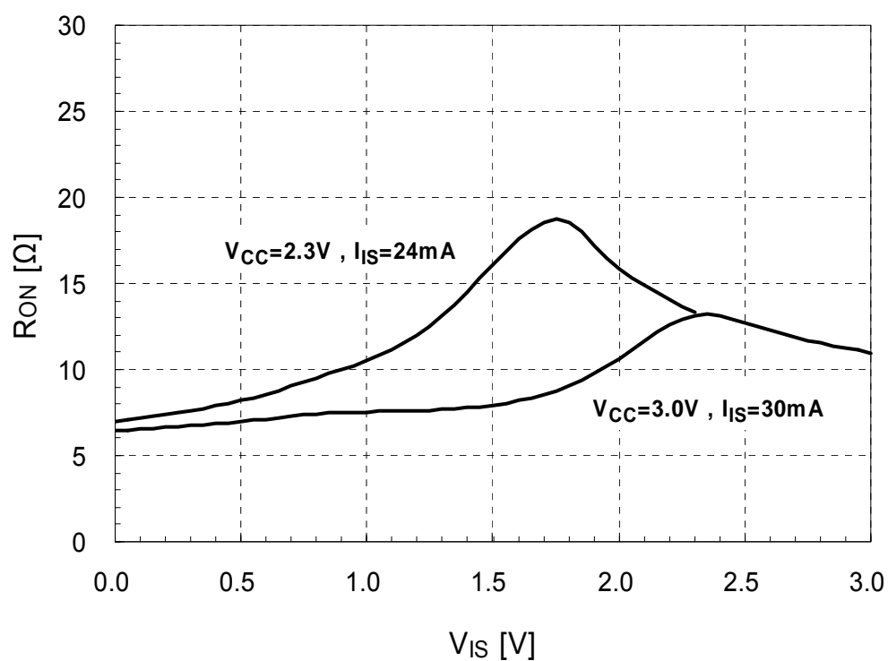
R_{ON} - V_{IS} Characteristic (typ.) T_a=25^\circ\text{C}
