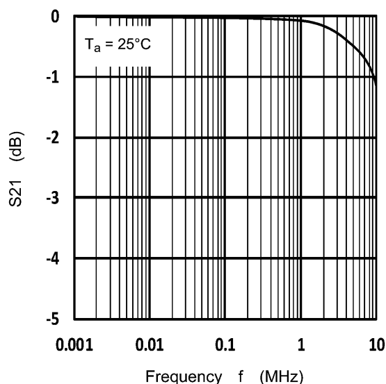
Fig. 10.1 S_{21} - f
