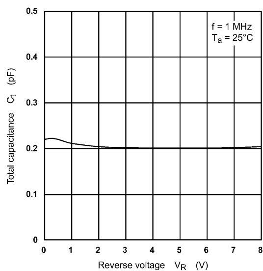
Fig. 8.3 C_t - V_R
