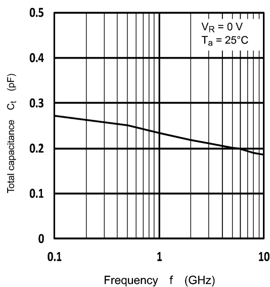
Fig. 8.4 C_t - f
