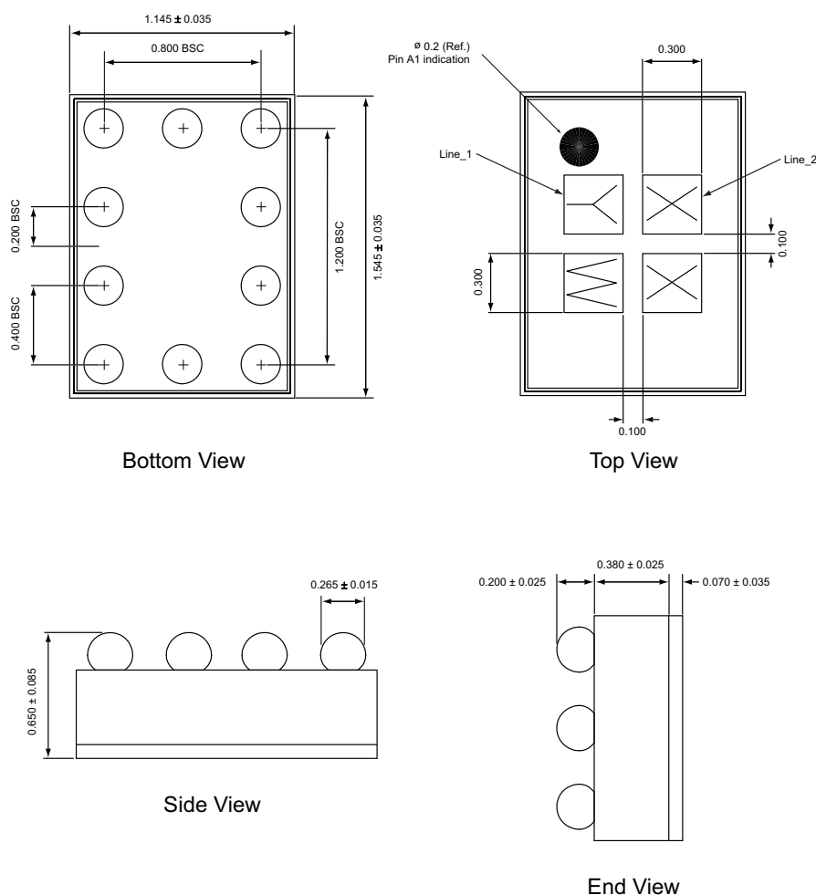
WLCSP-10
